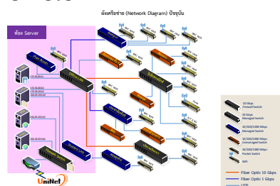
ผังเครือข่ายปัจจุบัน
